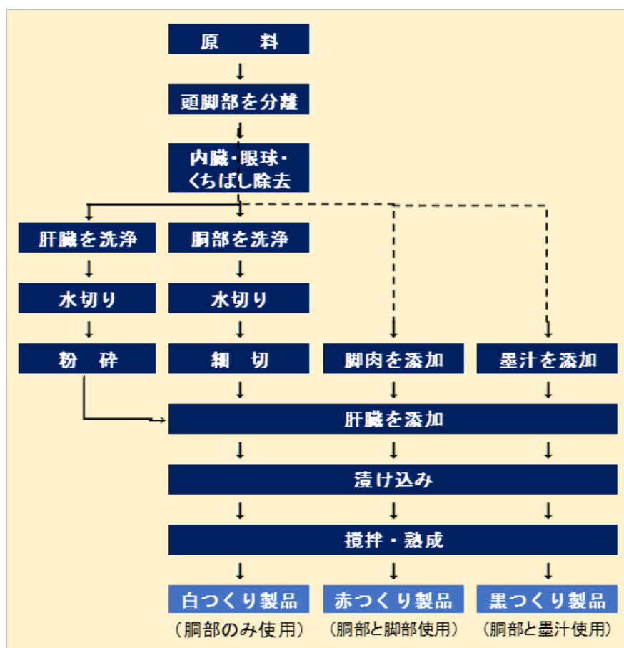
図2 イカ塩辛の製法
