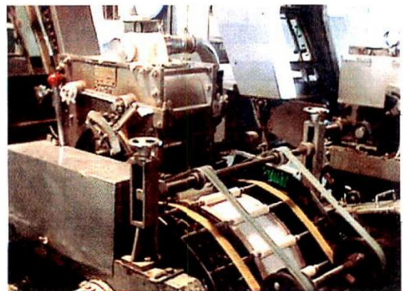
写真2 成形工程 (株)かね貞提供
